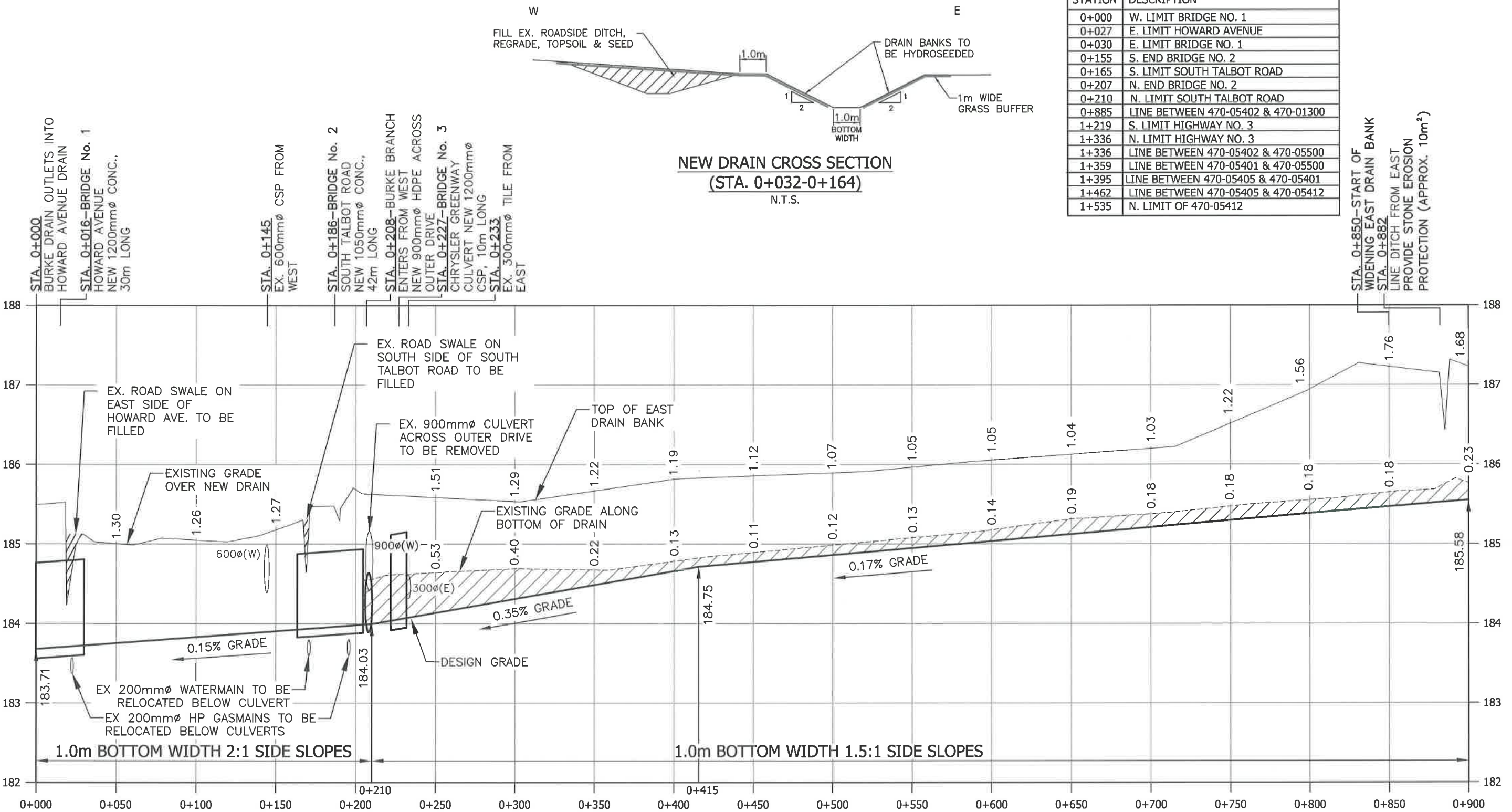
PROFILE 1 STA. 0+000 TO 0+900
